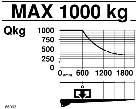
Belastungsdiagramm
